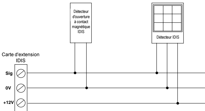
Figure 27. Raccordement d'une simple liaison IDIS
