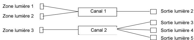
Figure 49. Canaux de commande d'éclairage
