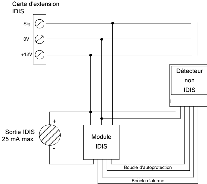
Figure 30. Utilisation du module universel IDIS
