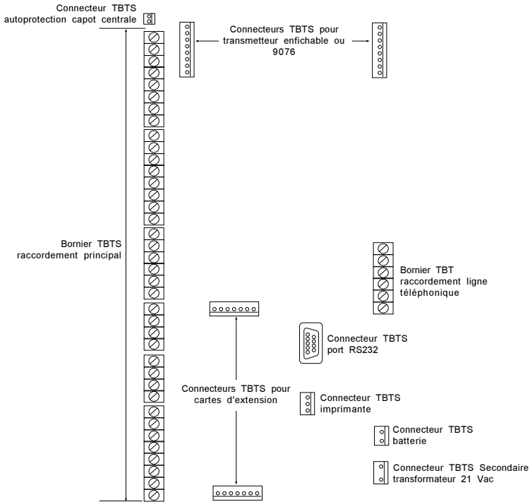
Figure 55. Connecteurs TBT et TBTS
