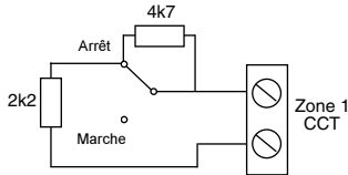
Figure 18. Contact à clé impulsionnel
