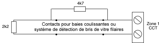
Figure 14. Connexion sur zone ZFS des contacts pour baies coulissantes ou systèmes de détection de bris de vitre filaires.
