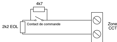
Figure 22. Câblage d'une zone pour la commande d'un système d'éclairage
