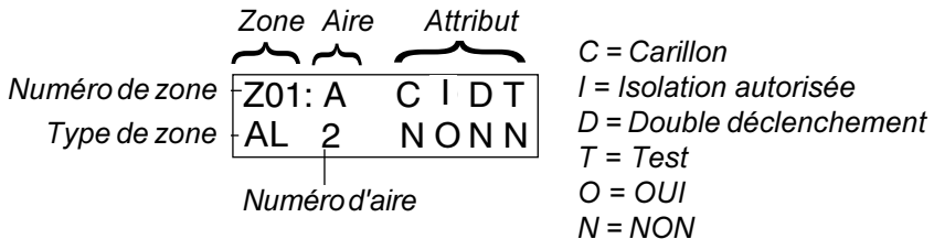
Figure 53. Affichage des zones pour le menu 32
