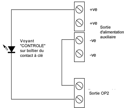
Figure 21. Raccordement d'un voyant "CONTROLE" sur un boîtier avec contact à clé
