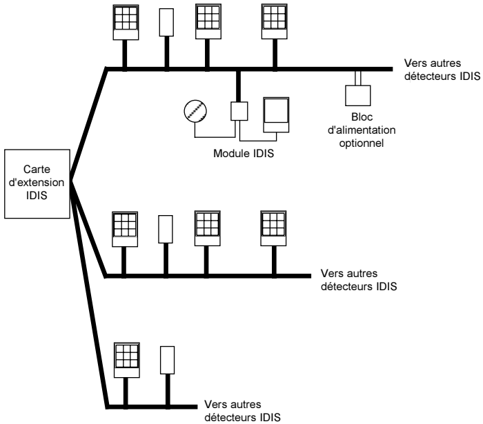
Figure 25. Configuration en "étoile"
