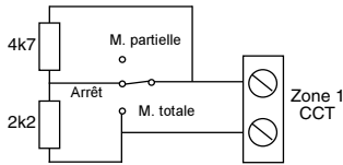
Figure 19. Contact à clé 3 positions Marche Totale / Partielle
