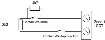
Figure 11. Raccordement d'un contact d'alarme unique avec autoprotection
