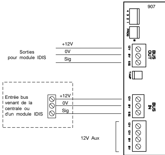
Figure 32. Utilisation d'un LIM IDIS 907
