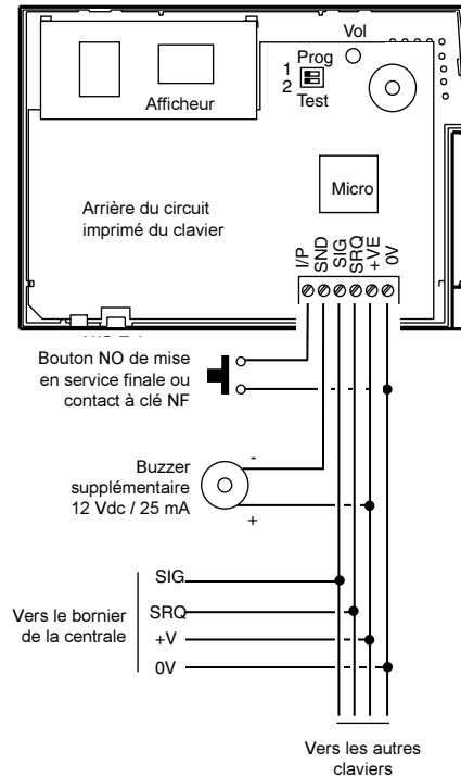
Figure 10. Raccordement d'un clavier 931
