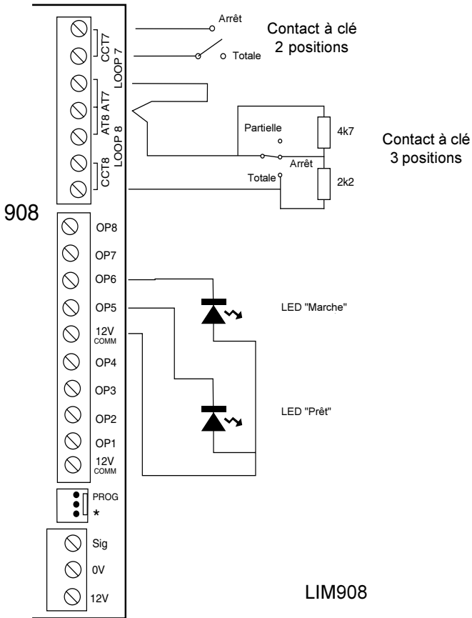
Figure 33. Câblage d'un boîtier à clé sur une zone IDIS
