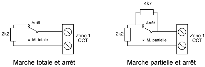
Figure 17. Contact à clé 2 positions M/A
