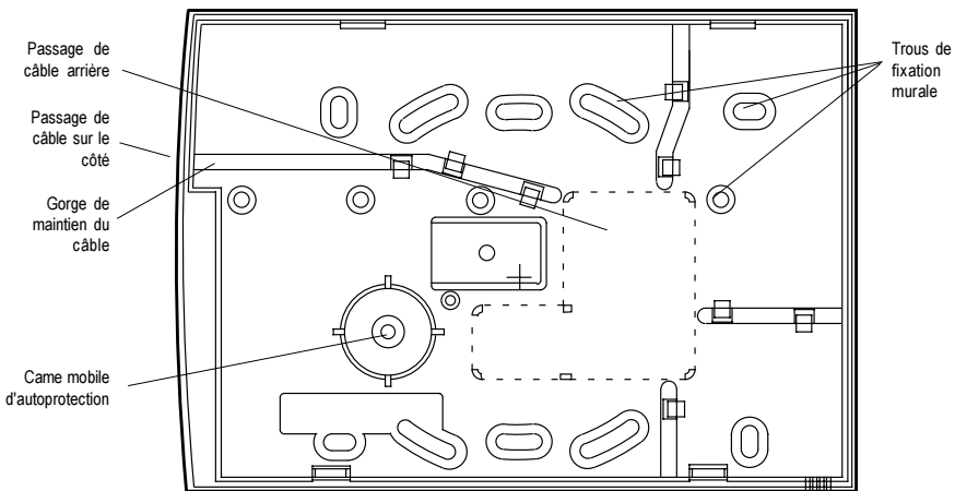
Figure 7. Embase du clavier 931
