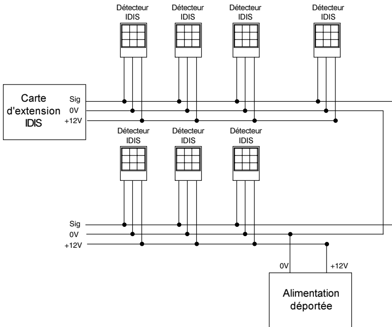
Figure 61. Emplacement de l'alimentation déportée
