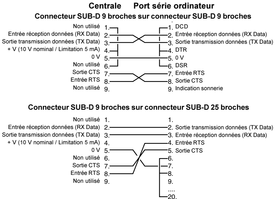
Figure 60. Signaux présents sur le connecteur série
