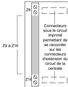
Figure 15. Carte d'extension ZFS (référence 943UK-00)
